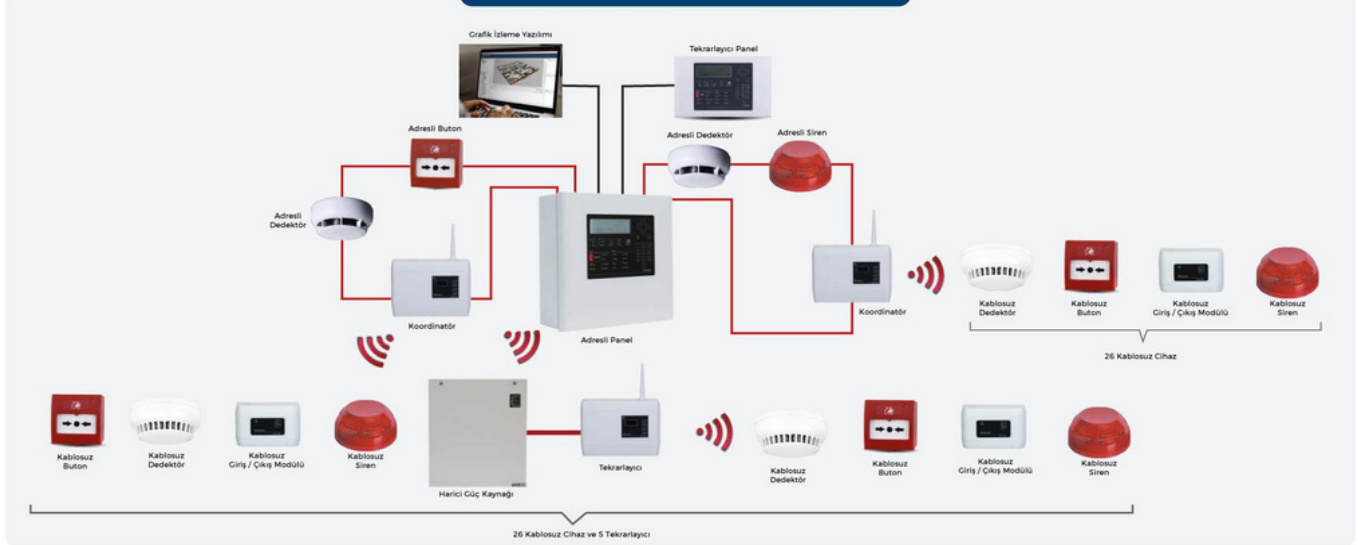
Kablosuz Adresli Yangın Sistem Şeması
