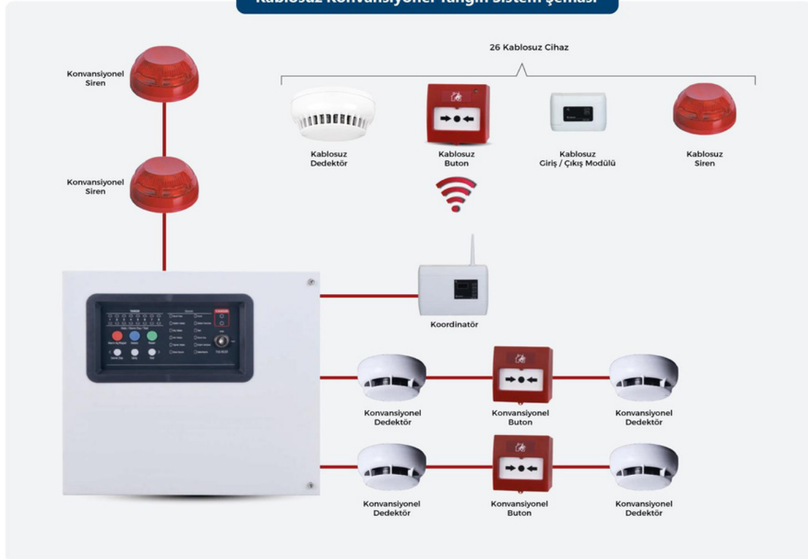
Kablosuz Konvansiyonel Yangın Sistem Şeması
